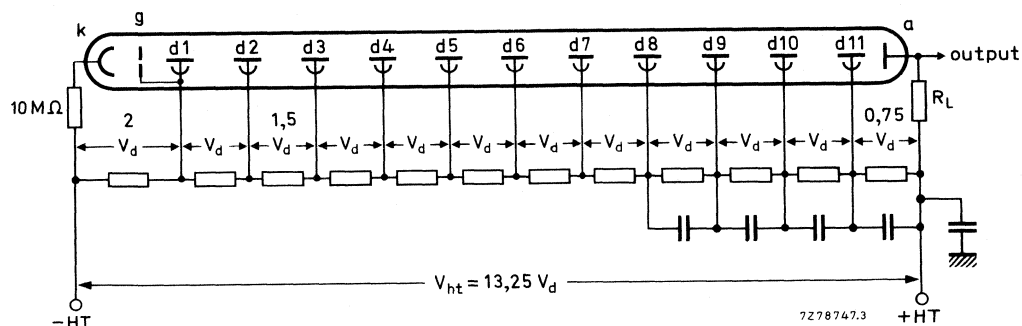
Fig. 2 Voltage divider A.
