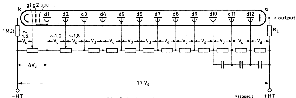
Fig. 2 Voltage divider type A.
