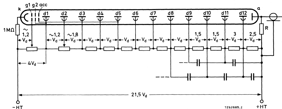
Fig. 4 Voltage divider type B'.
