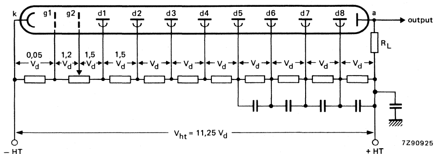
Fig. 2 Voltage divider A.
