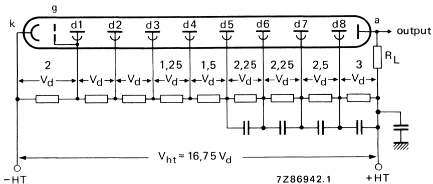
Fig. 3 Voltage divider B.
