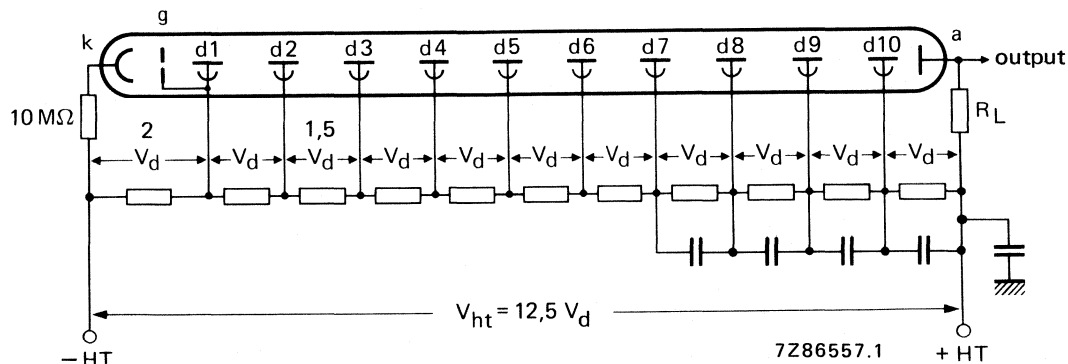
Fig. 2 Voltage divider A.
