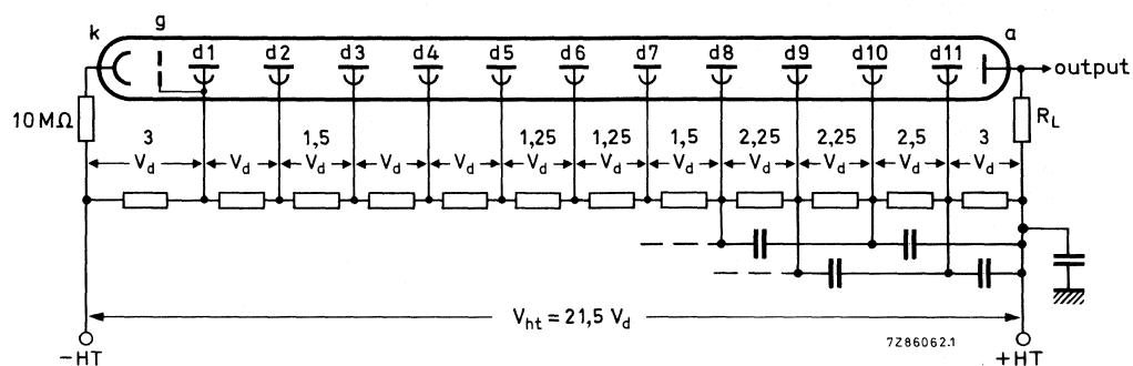
Fig. 3 Voltage divider B.
