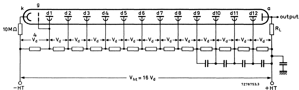
Fig. 2 Voltage divider A.
