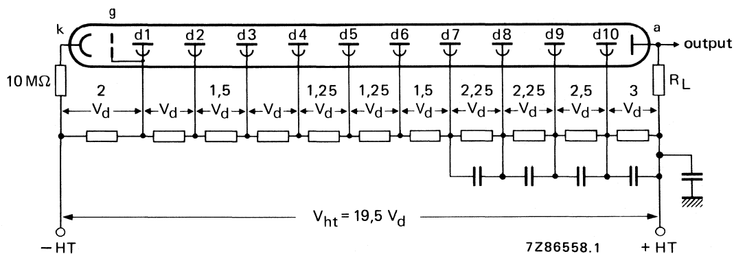
Fig. 3 Voltage divider B.
