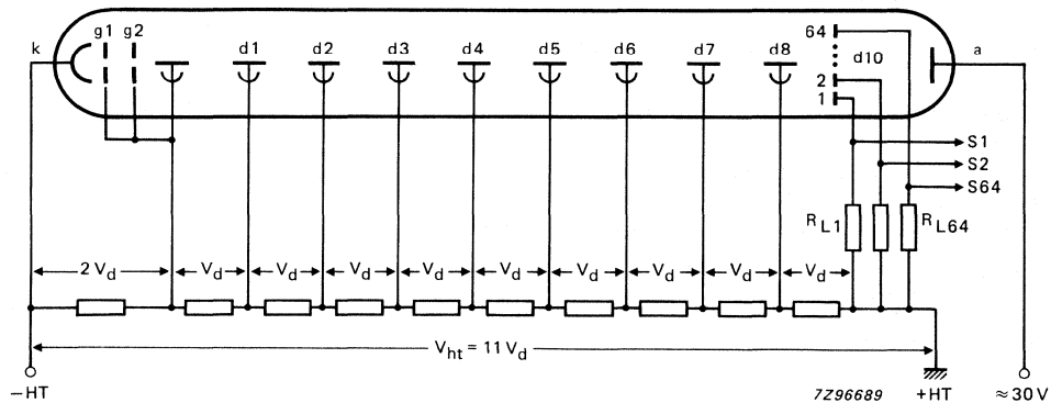
Fig. 1 Voltage divider.
